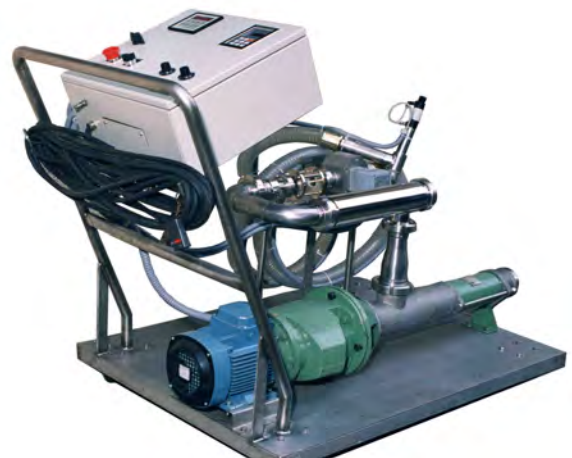
Equipo dosificador con bomba tipo mono, contador de turbina y programador
