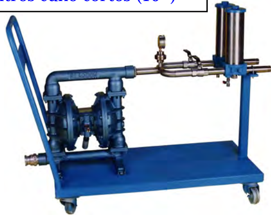
Equipo de trasiego con bomba de membranas de aluminio-teflón de 1 1/2" y dos filtros cunco cortos (10")
